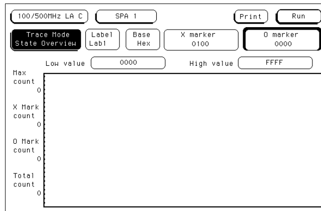
Default SPA Menu
